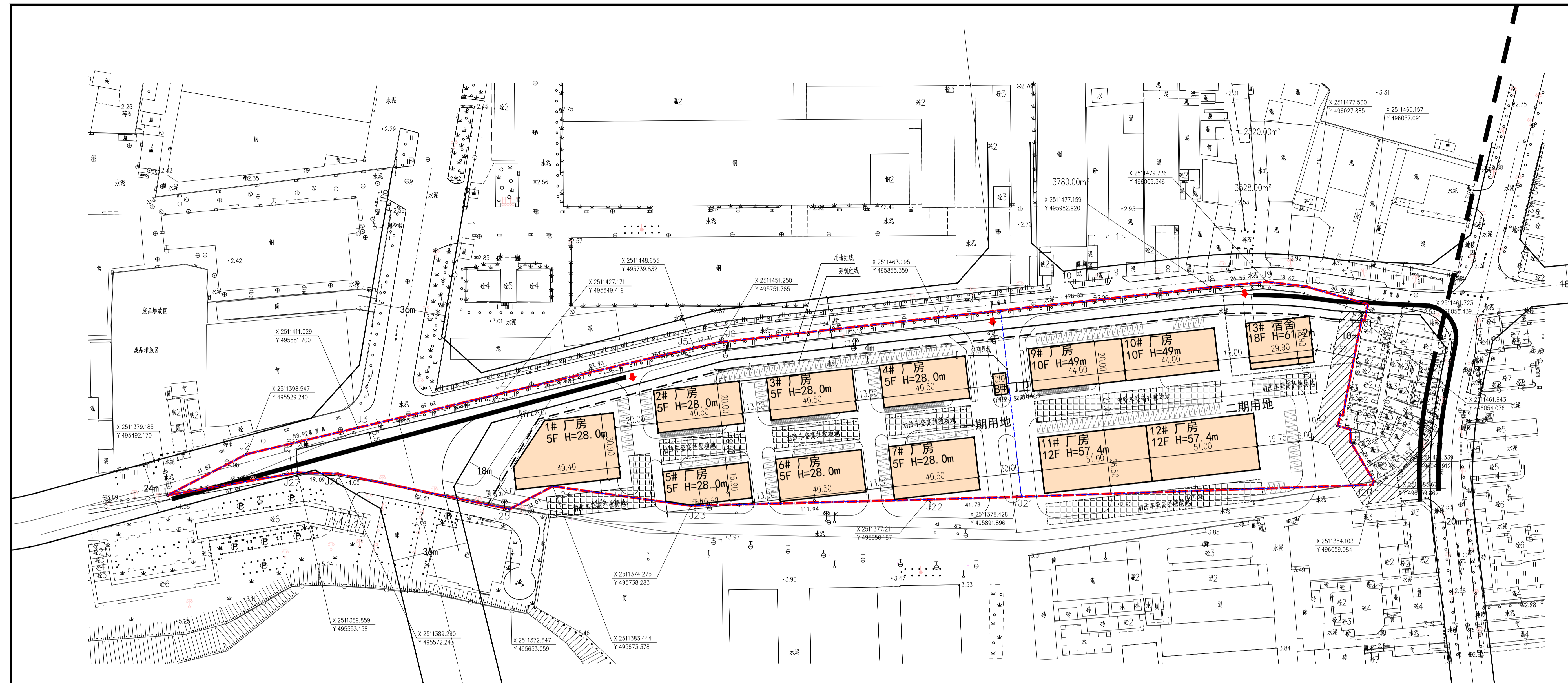
总平面图 1:1000
